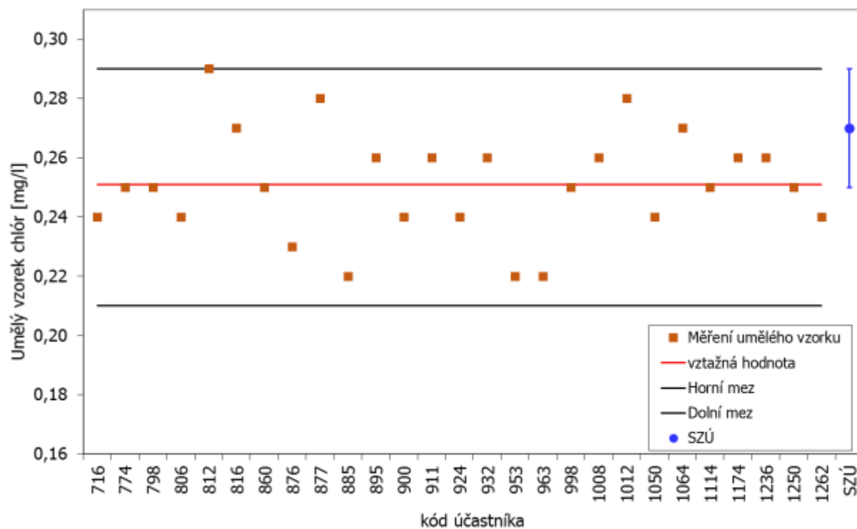
Graf 1: Stanovení volného chloru v uměle připraveném vzorku
