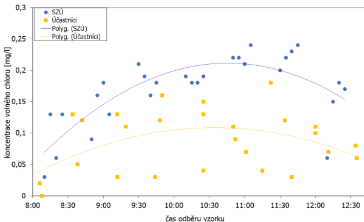
Graf 2: Stanovení volného chloru v bazénové vodě
