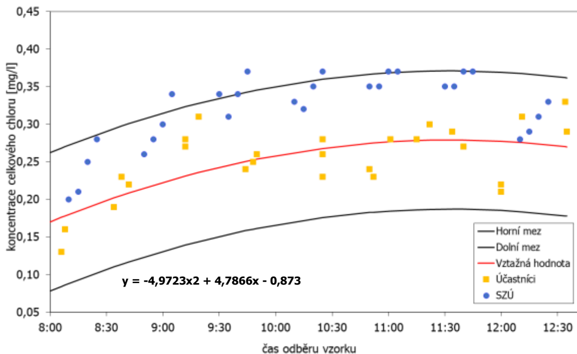
Graf 3/B: Stanovení celkového chloru v bazénové vodě, upraven dle uvedené polynomické rovnice
