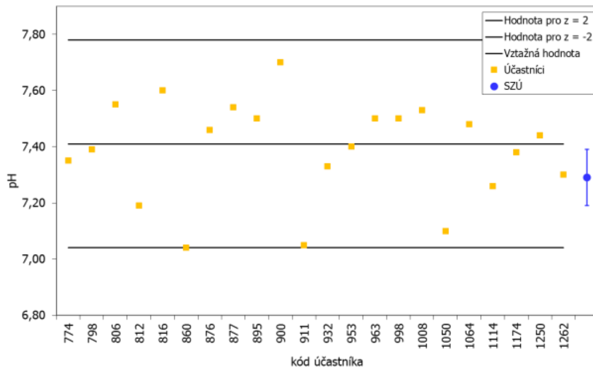
Graf 5: Stanovení pH v bazénové vodě
