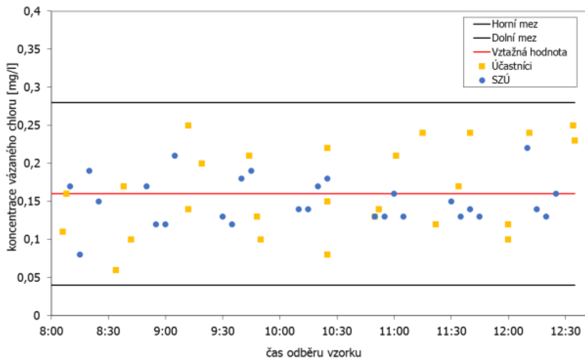
Graf 4: Stanovení vázaného chloru v bazénové vodě
